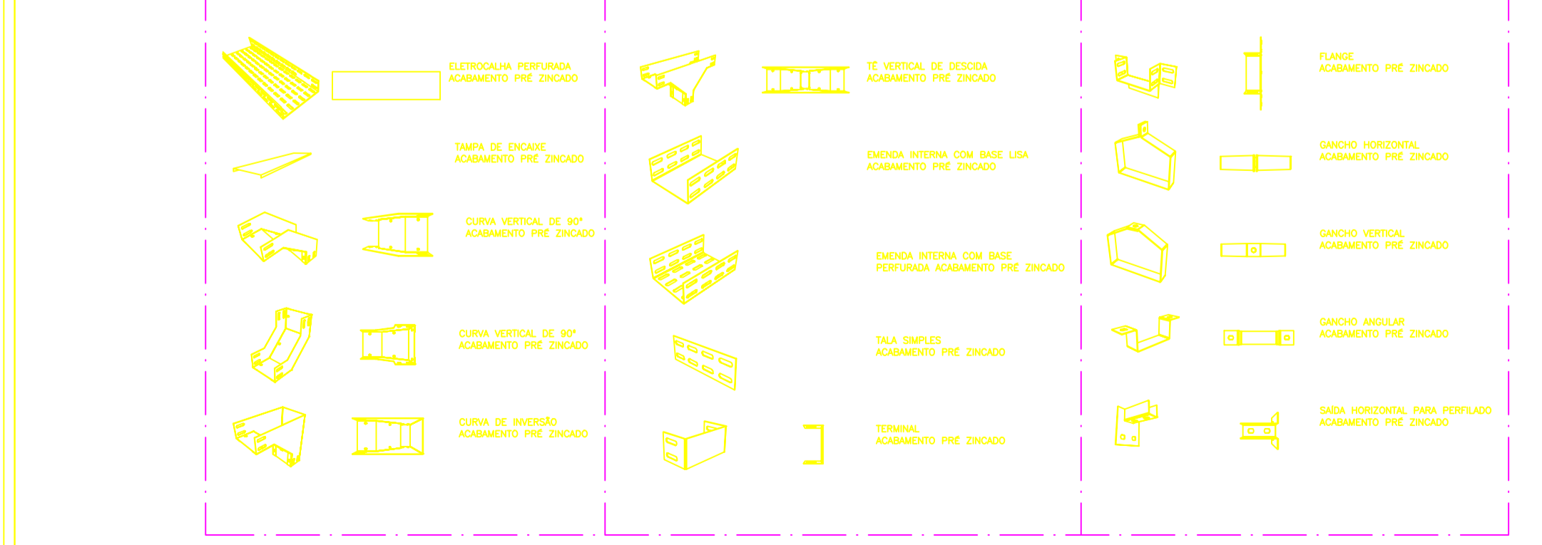
06 DETALHE 03 - ACESSÓRIOS E CONEXÕES ESCALA: S/ESC.
